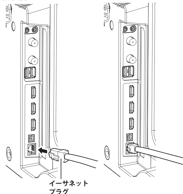
接続例
